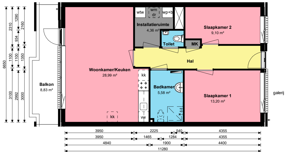
1e verdieping
