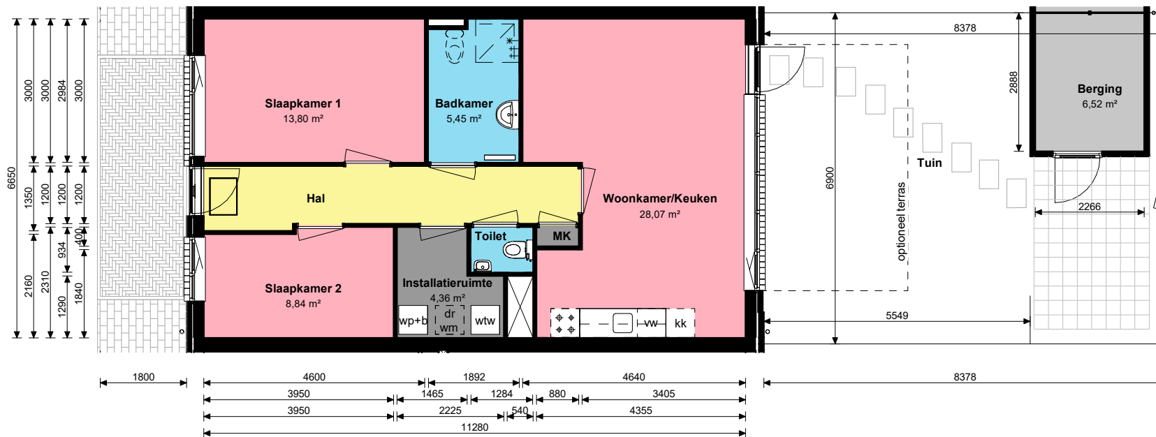
Begane grond
